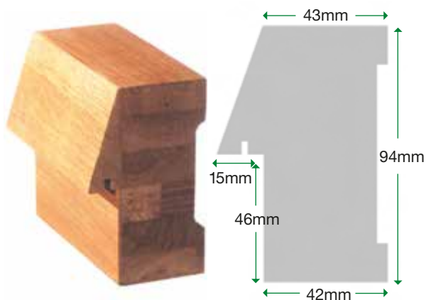
FRAME JAMB OR HEAD
